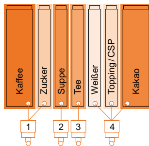
Variante 7403 7 Produktbehälter, 4 Mixereinheiten
